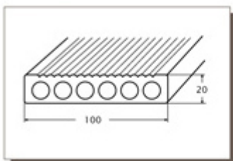
ontelorakenne
