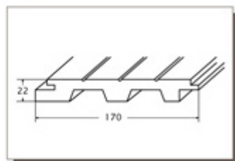
pontattu lauta
