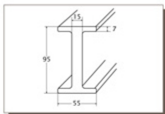
kaksisuuntainen palkki
